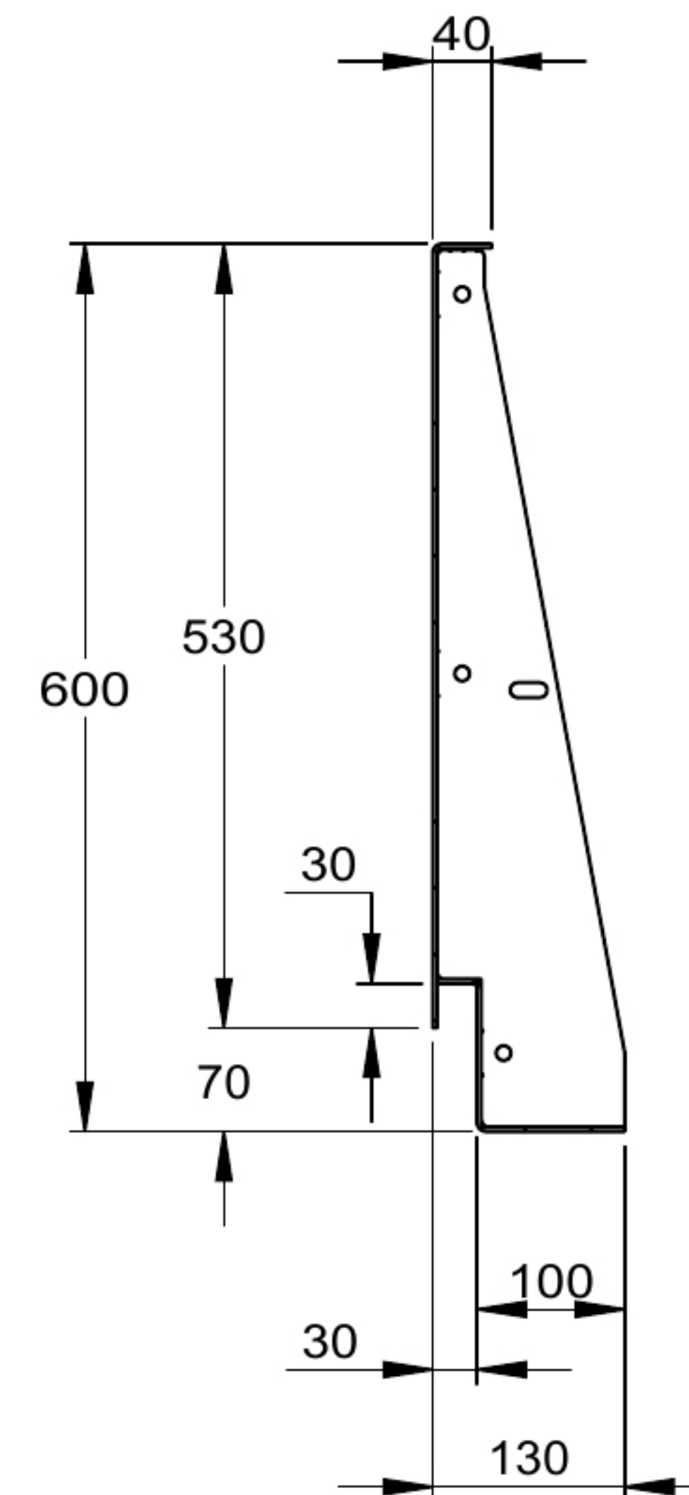
SECTION A-A
