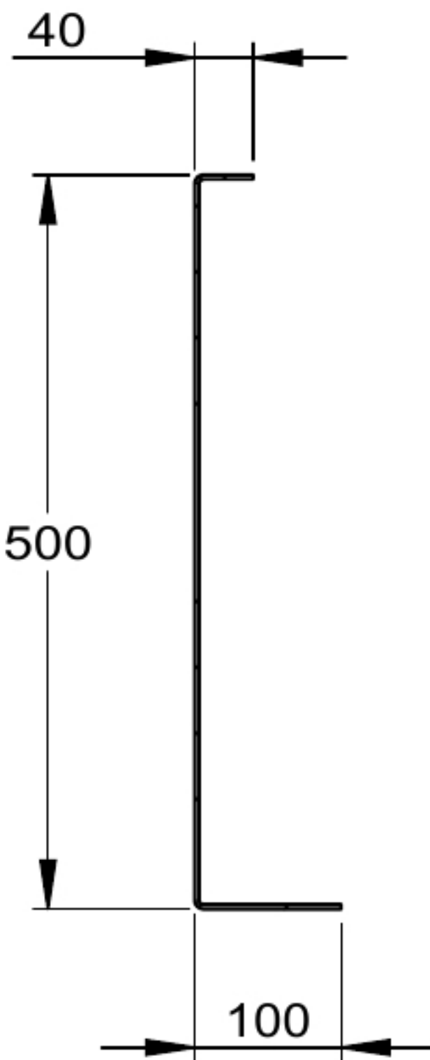
SECTION A-A
